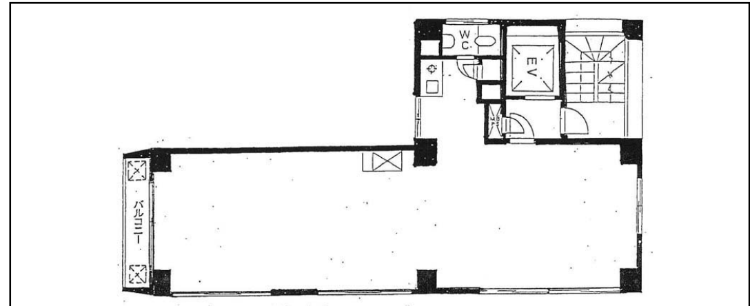
5階平面図
